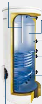
WSTB 300 C WSTB 160-200 WSTB 120 O
