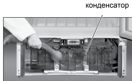
конденсатор ХТ-1006-XXX
