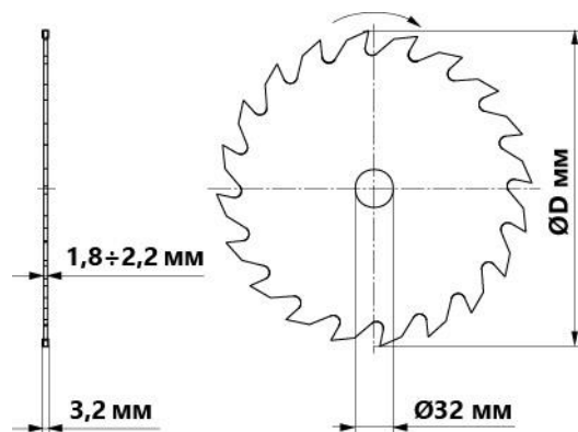
Рисунок 15. Диск пильный
