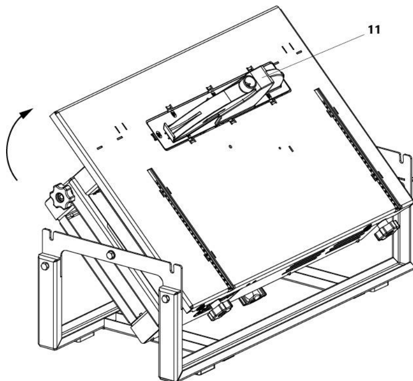
Рисунок 2. Поворот станка с операции пиления на строгание 11 – кожу
