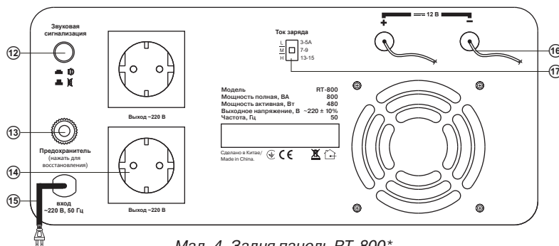
Мал. 4. Задня панель RT-800*
